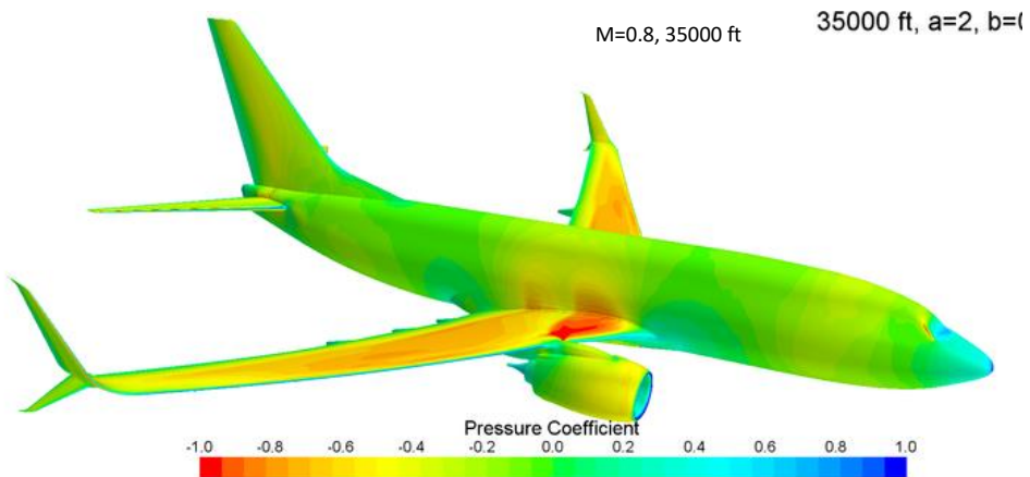
Figuur 4 Verschildrukverdeling op de B737 MAX uitgedrukt als drukcoëfficiënt (“pressure coefficient”)
