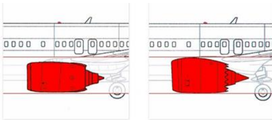
Figuur 3 Motorgondels van links de B737 NG en B737 MAX
